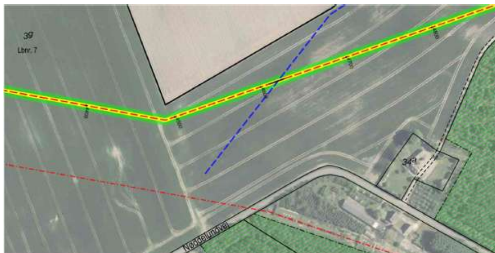
Figur 5. Udklip fra ansøgning. Matrikelnr. 3g Sahl By, Sahl. Styret underboring af "Tilløb til Skibelund Bæk 2" på cirka 12 meter. Kort sort streg angiver start- og slutpunkt for den styrede underboring. Blå stiplede linje angiver vandløbet.
