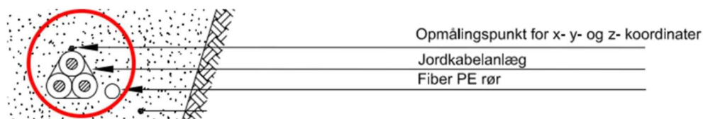
Figur 1. Principskitse af underboring med rødt foringsrør indeholdende 3 kabler og et 40 mm rør.
