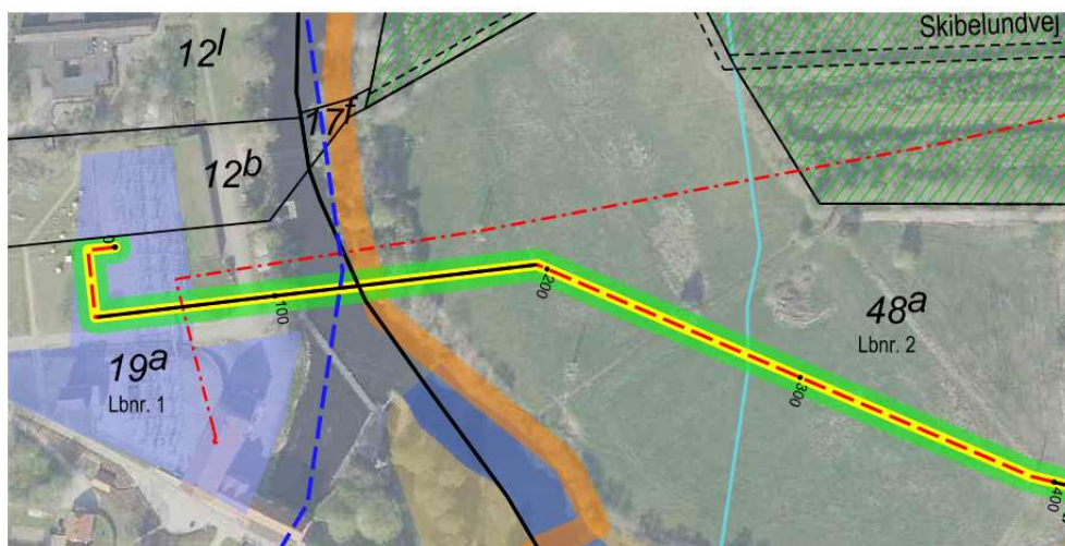
Figur 7. Udklip fra ansøgning. Matrikel nr. 48a Sahl By, Sahl og 19a Tange By, Højbjerg. Styret underboring af Gudenåen. Sort streg angiver start- og slutpunkt for den styrede underboring. Den blå stiplede linje angiver vandløbet. Underboringen forventes at blive ca. 170 m.
